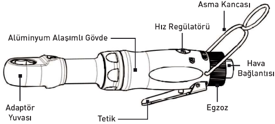
Asma Kancası
